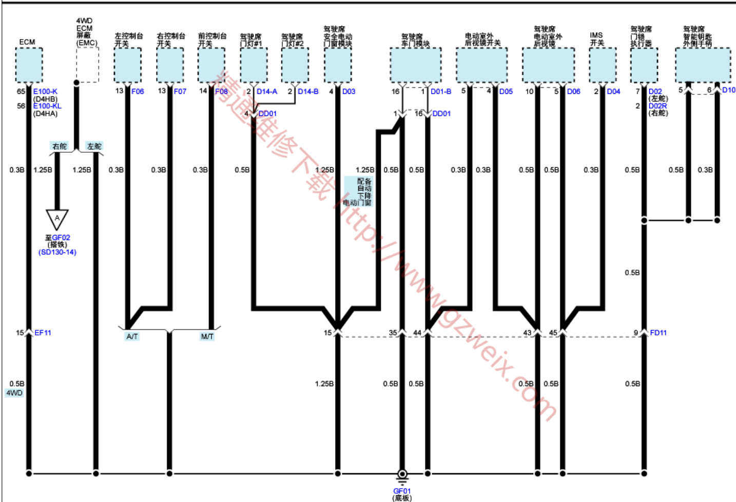
搭铁分布(12)
